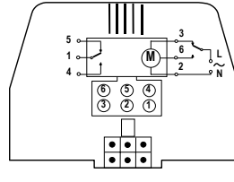
Abb. 8: VC-Stellglied mit Molex™ Anschluss für SPDT-Regler
